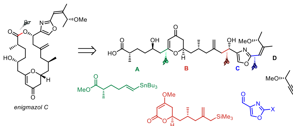
Obrázek 2. Retrosyntéza Enigmazolu C
