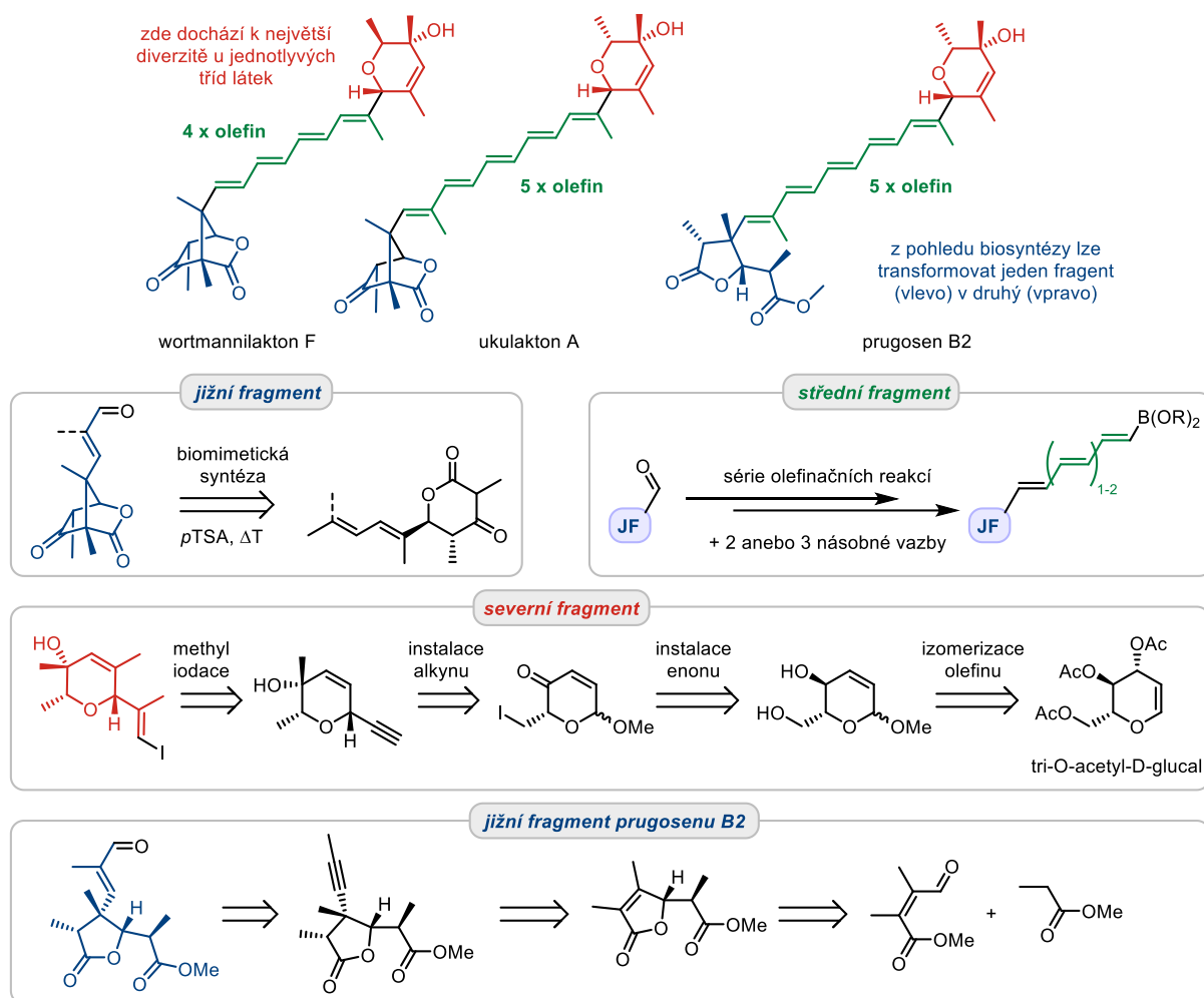
Obrázek 2. Struktury wortmannilaktonů a prugosenů.
